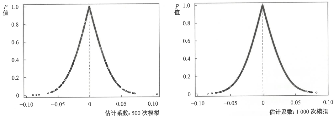
图3 安慰剂检验
